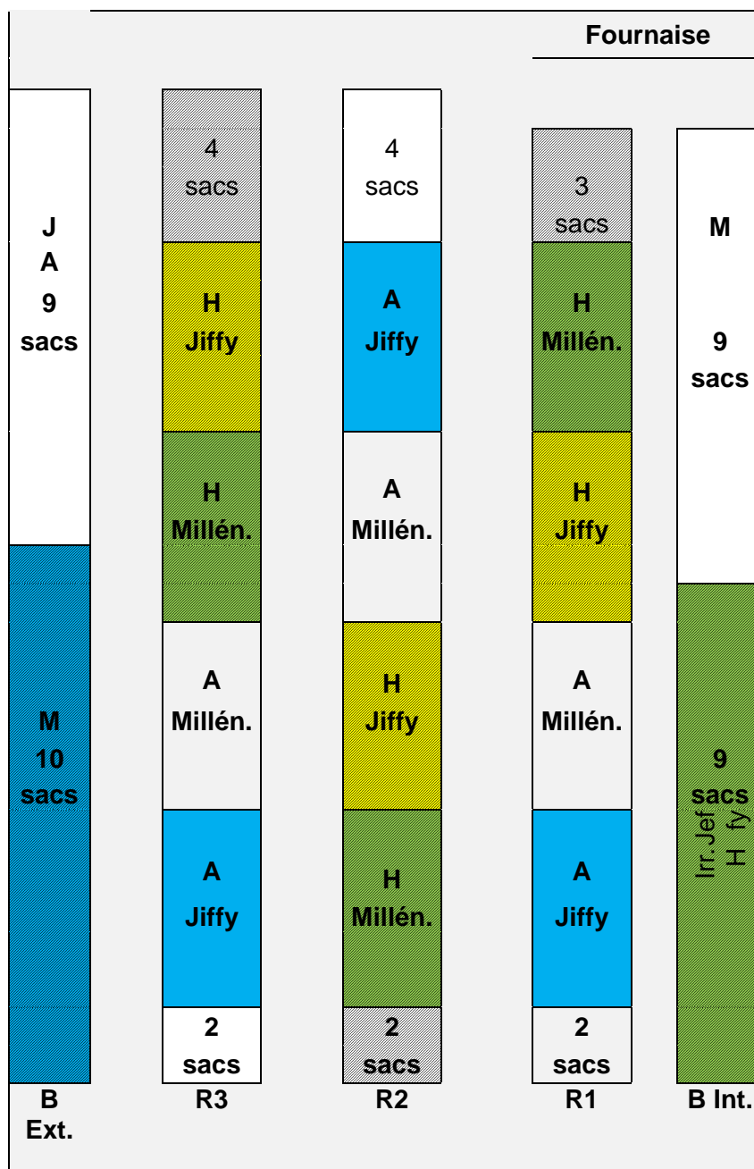
Figure 3. Schémas du dispositif expérimental Tomate 2010 serre K2.
