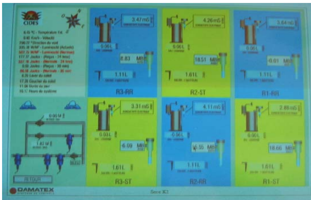
Figure 2. Interface graphique des systèmes d'irrigation (Bleu= Aérée, Jaune= Humide).
